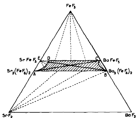
FIG. 4. Le système \text{BaF}_2 - \text{SrF}_2 - \text{FeF}_3 à 700^\circ\text{C} .
